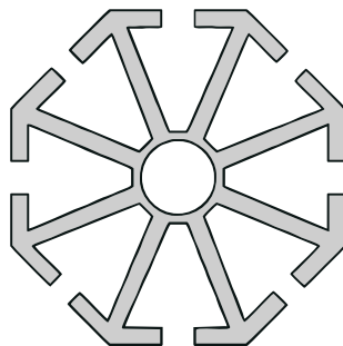
40x40 ALU-8 kahdeksalla uralla 45 asteen jako. Erinomainen yksinseisovana monitoimi jalkana. M10 kierre päissä. Musta ulverimaalaus mahdollinen.
