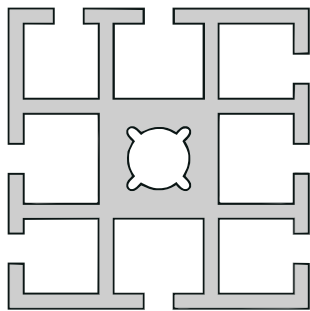
40x40 ALU-4 tolppa 3, 2, 2, 1 uraisena. Profiilin toimintaa voi muuttaa kääntämällä sen. M10 kierteet päädyissä. Anodisoitu ja siksi säänkestävä.
